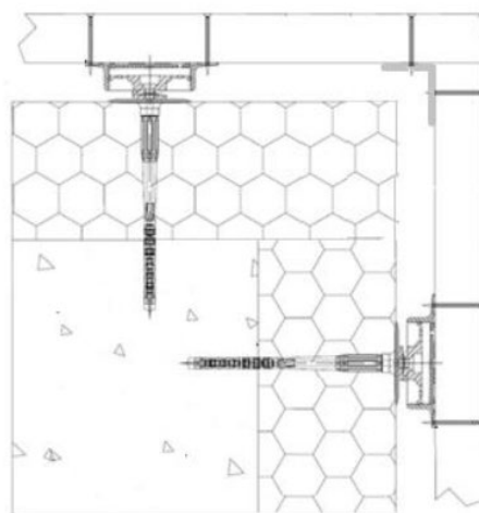
Figure 5 : traitement des angles sortants, avec une cornière rapportée dans l'angle des plaques de plâtre
