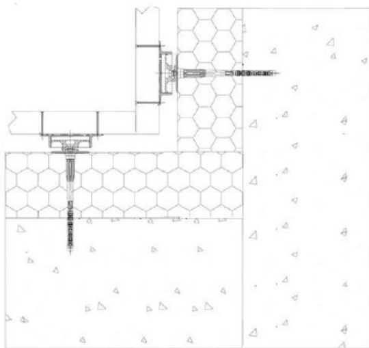
Figure 4 : traitement des angles rentrants
