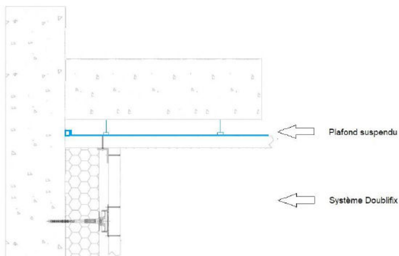
Figure 6 – Jonction des doublages sous les plafonds suspendus
