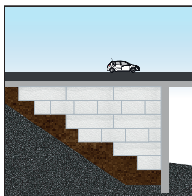
Réduction des poussées sur les ouvrages d'art
