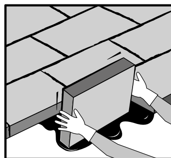
Pose des panneaux : les deux bords du panneau sont trempés dans l'EAC.
