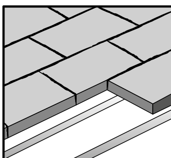
Figure 5 - Sens de pose des panneaux en verre cellulaire sur TAN
