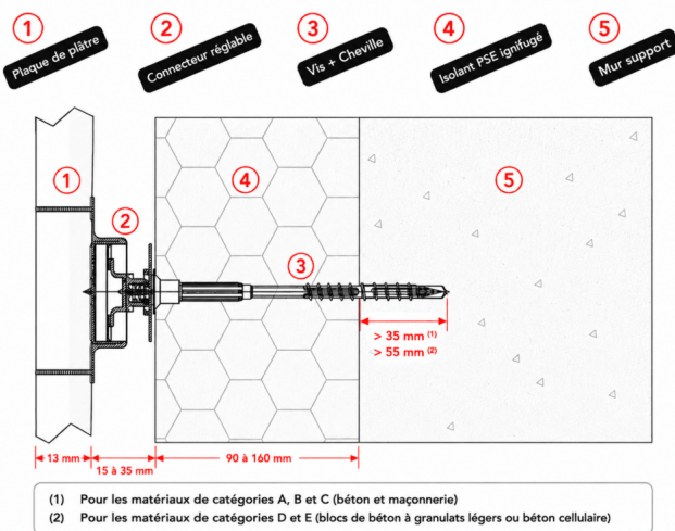
Schéma de composition du Système Doublifix®
