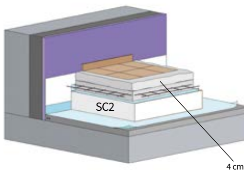
Isolation en pose scellée directe d'un carrelage sur forme avec treillis
