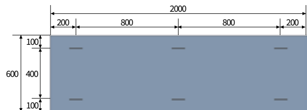
6 chevilles jusque 190 mm d'épaisseur
