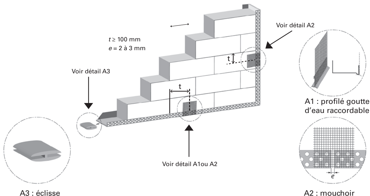
Figure 1 – Disposition des profils de départ et latéraux – Renforts aux jonctions entre profilés
