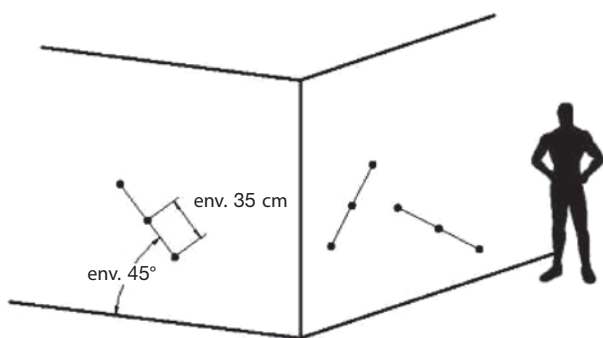
Figure 10 – Exemple d'emplacement des fixations mécaniques dans le support
