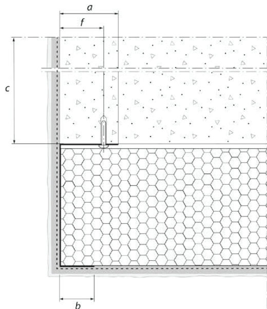
Figure B1.1 – Arrêt latéral en angle sortant variante 1 (recouvrement d'armatures ; coupe horizontale)
