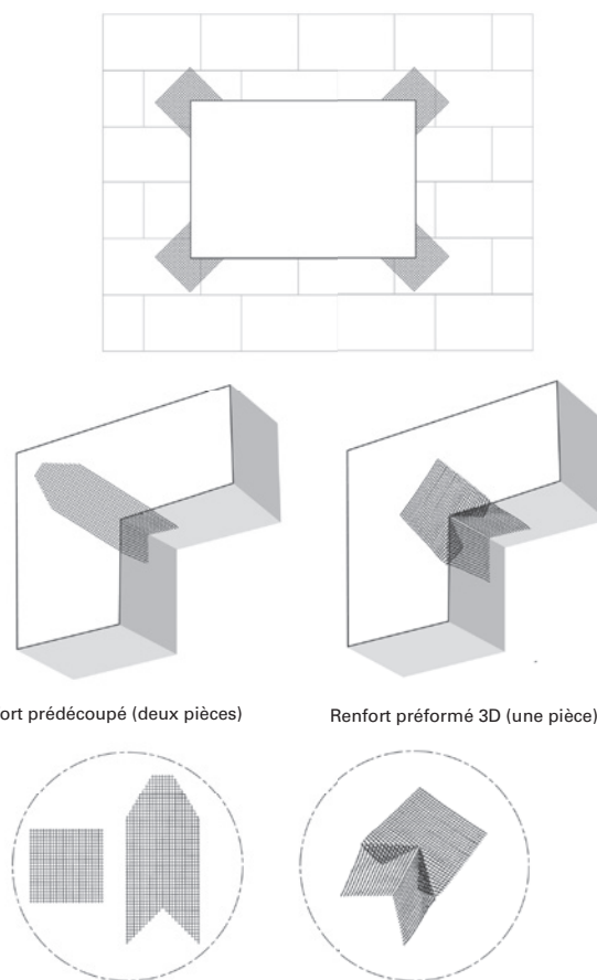
Figure 7 – Renforts aux angles des baies
