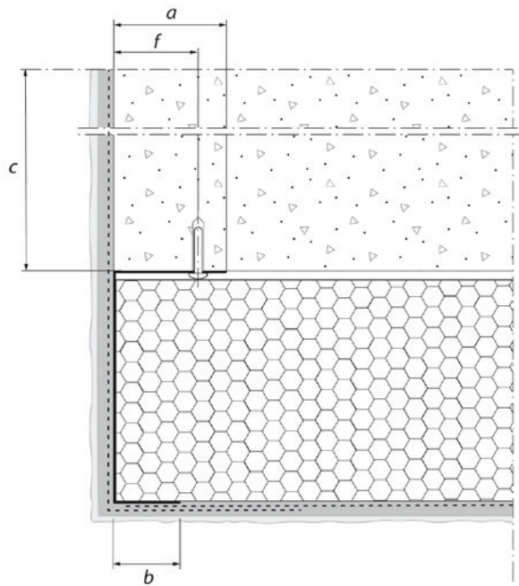
Profilé d'arrêt latéral perforé
