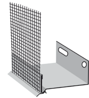
Profilé de départ avec profilé raccordable en face avant
