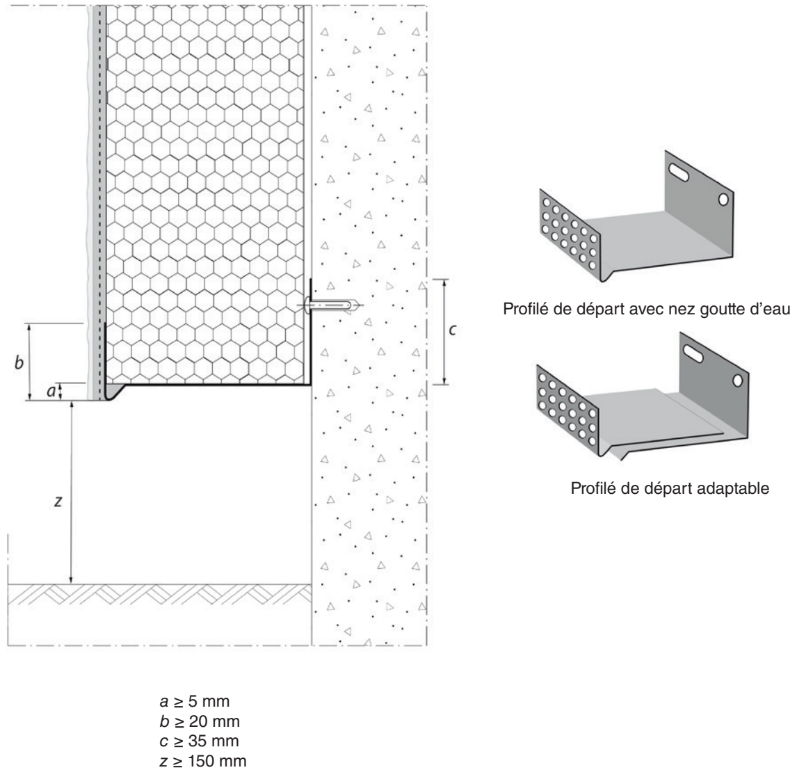
Figure A1.1 – Départ depuis le sol extérieur fini variante 1
