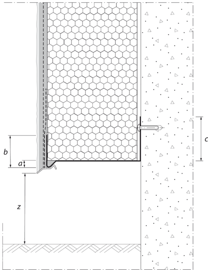
Profilé de départ avec profilé raccordable en face avant
