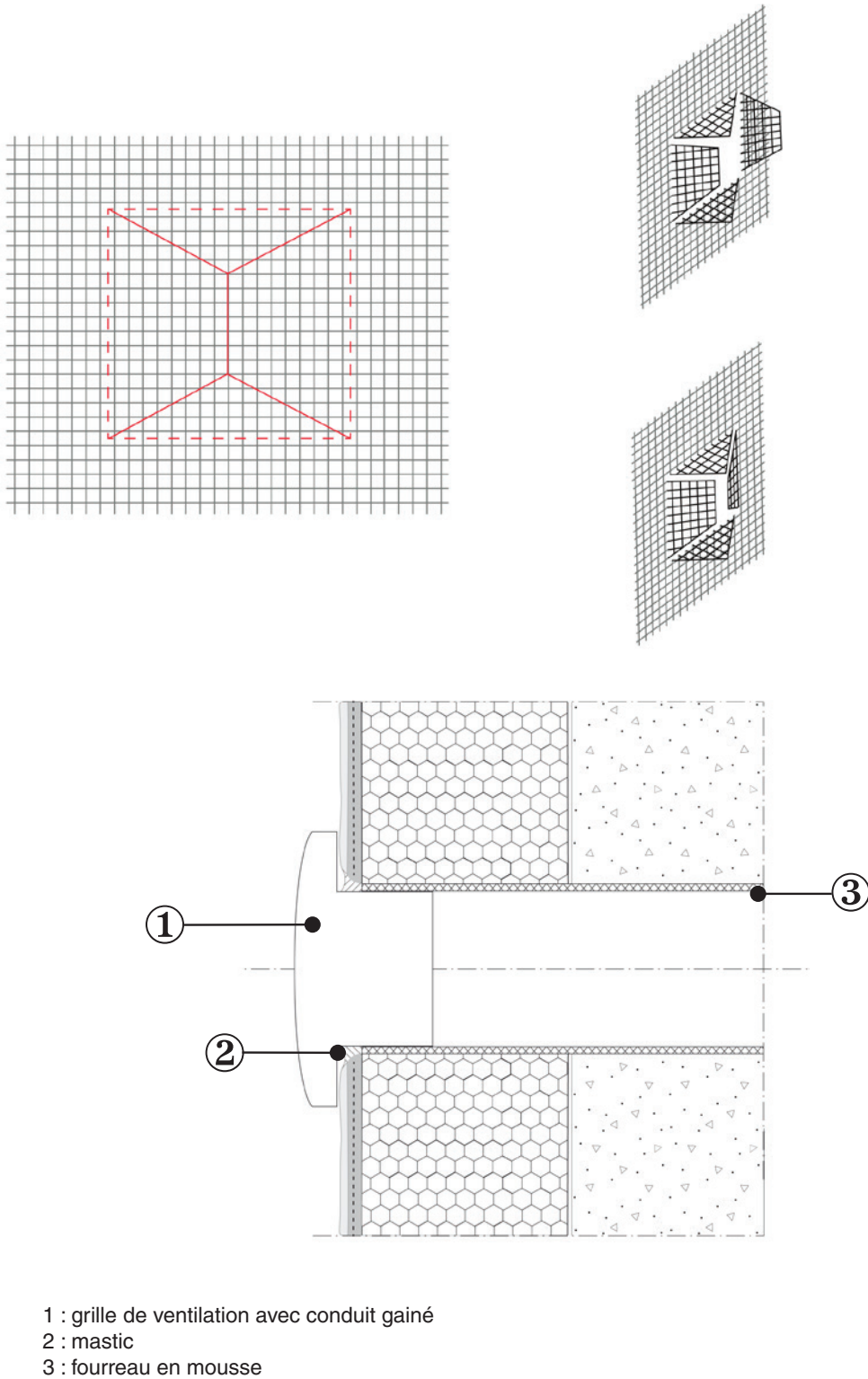
Figure F1 – Orifice de ventilation
